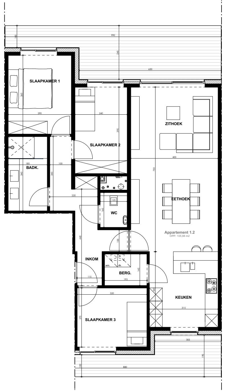
GRONDPLAN
